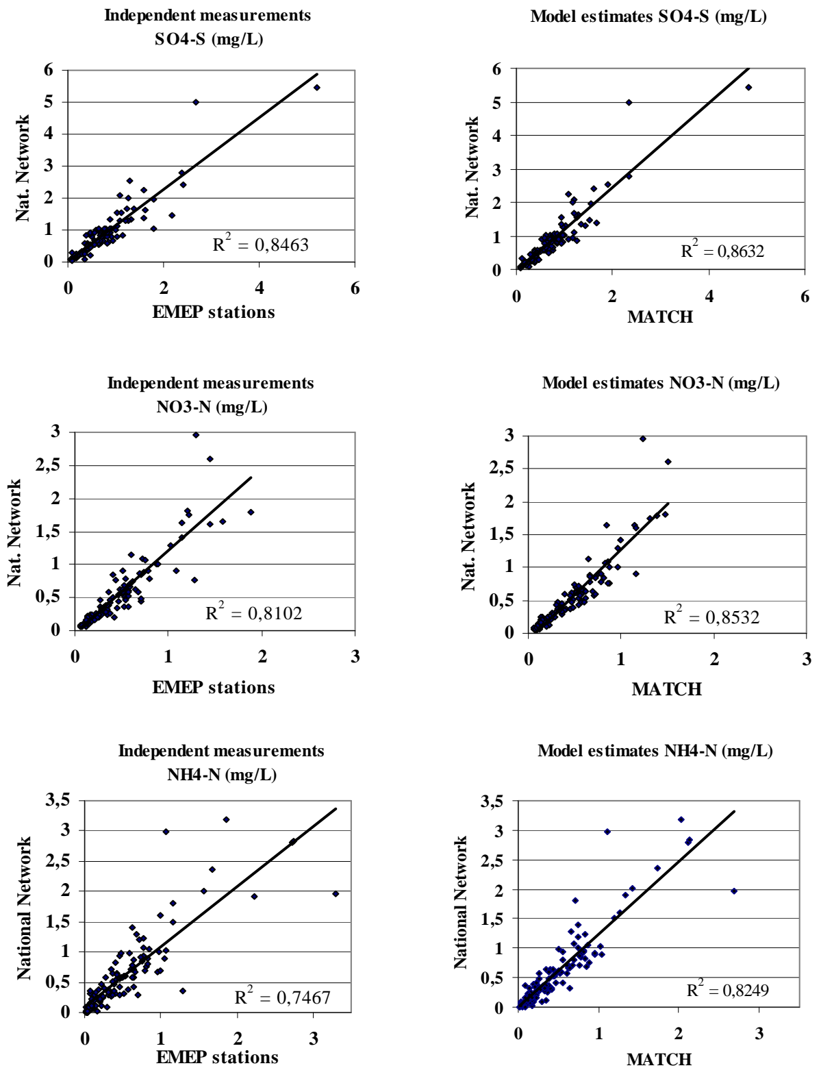
Figur 1. Spridningsdiagram som visar månadsvärden för halter i nederbörd ( SO_4 , NO_3 och NH_4 ) från 1994-1997 för tre platser: Vavihill, Aspvreten och Bredkålen, där EMEP- and LoN-stationer (National Network) är samlokaliserade. I vänstra kolumnen jämförs oberoende mätdata för EMEP och LoN. I högra kolumnen görs motsvarande jämförelse mellan MATCH-Sverige data och oberoende LoN(National Network)-data.
